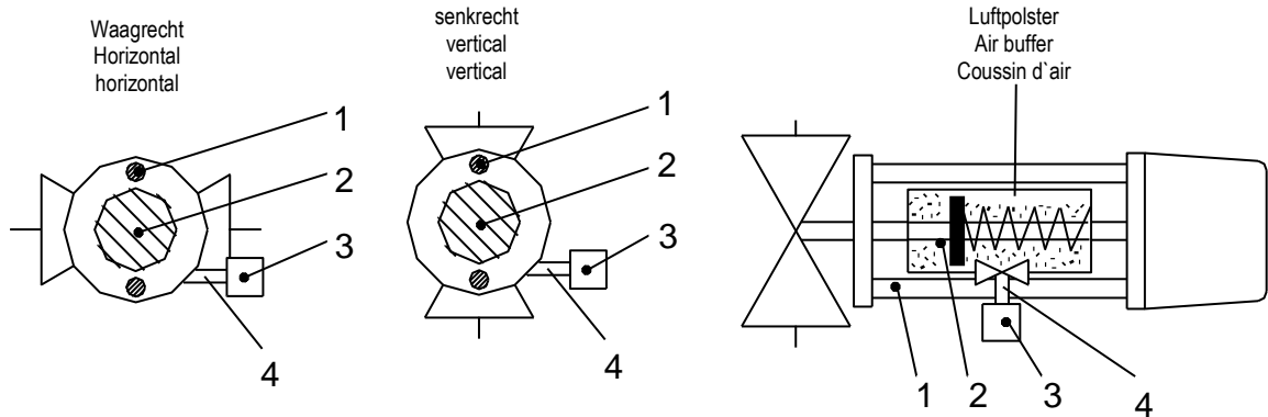
Bild 1 / figure 1 / photo 1: Einbaulage Schnellschlusseinrichtung waagerechter Einbau / mounting position emergency closing horizontally / position de montage vertical
