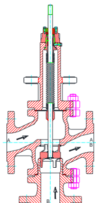
MV 5224 DN 20-100, PN 16 / 25 MV 5224 DN 20-150, PN 16 / 25
