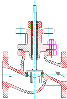
MV 5211 DN 15-65, PN 16-40 MV 5311 DN 15-65, PN 16-40
