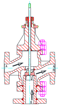
MV 5221 DN 25-100, PN 63-160 MV 5321 DN 25-100, PN 63-160
