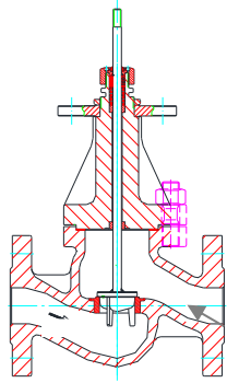
MV 5211 DN 15-100, PN 63-160 MV 5311 DN 15-100, PN 63-160
