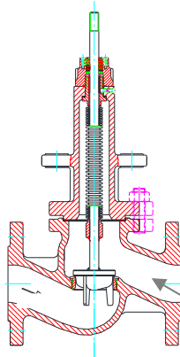
MV 5214 DN 15-100, PN 16 / 25 MV 5314 DN 15-150, PN 16 / 25
